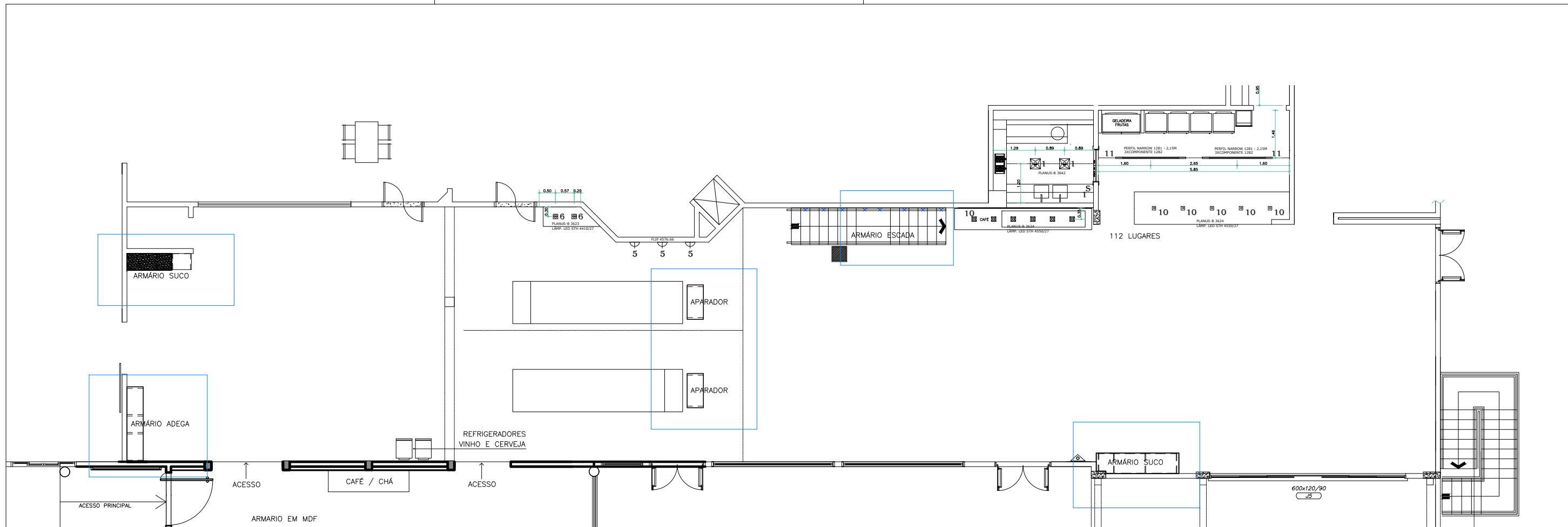
Arquitetonico - Restaurante Planta Baixa Escala 1/125
