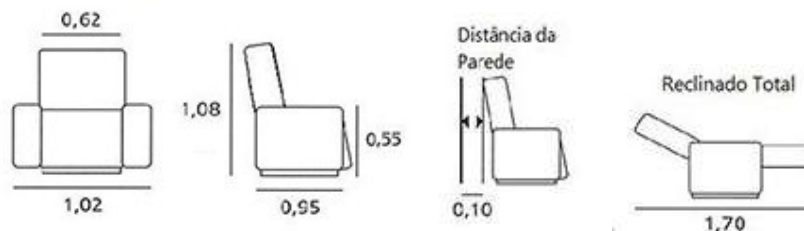
Figura 01 – Dimensões da poltrona em metros
