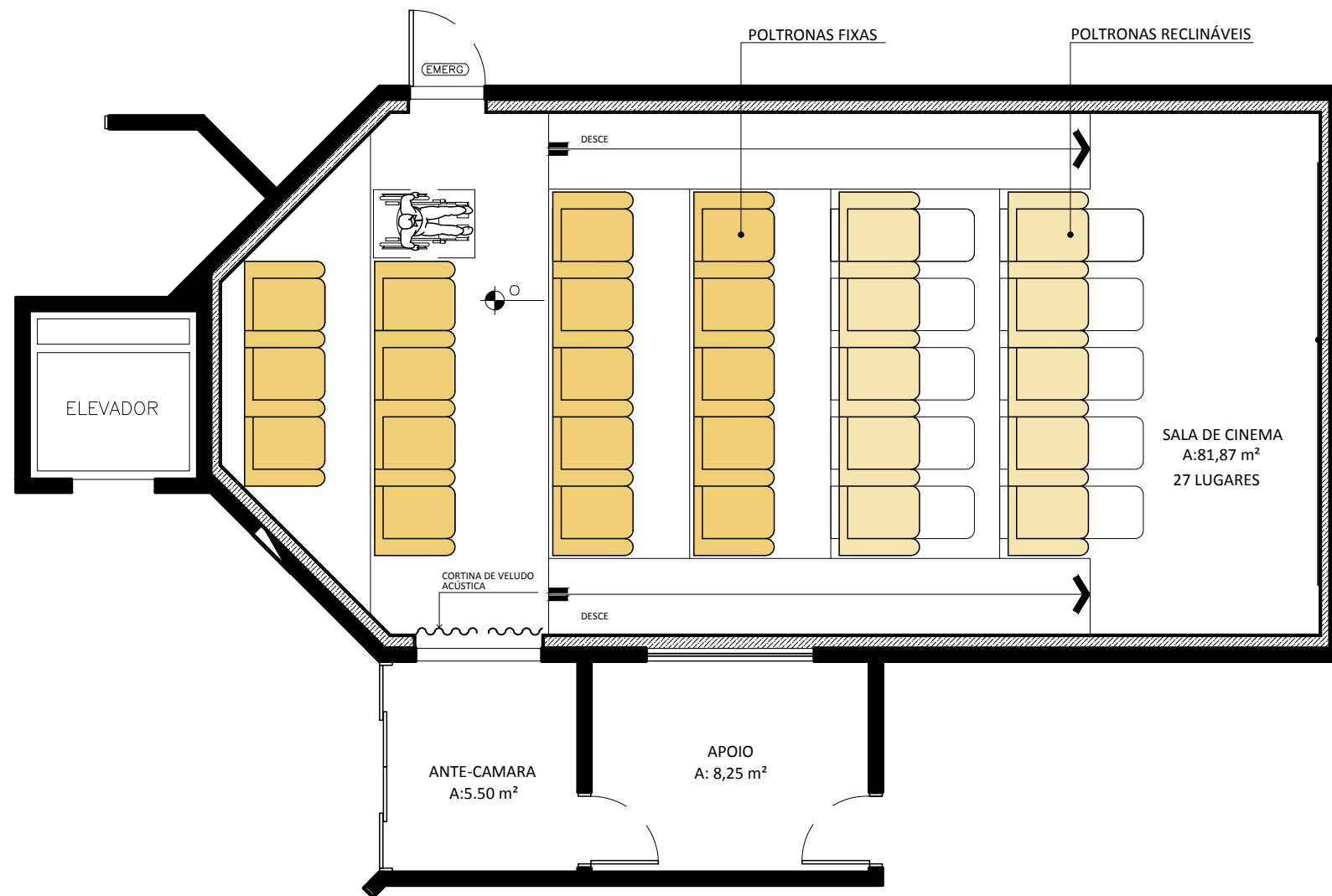
Arquitetónico - Cinema Planta layout Cinema Escala 1/75
