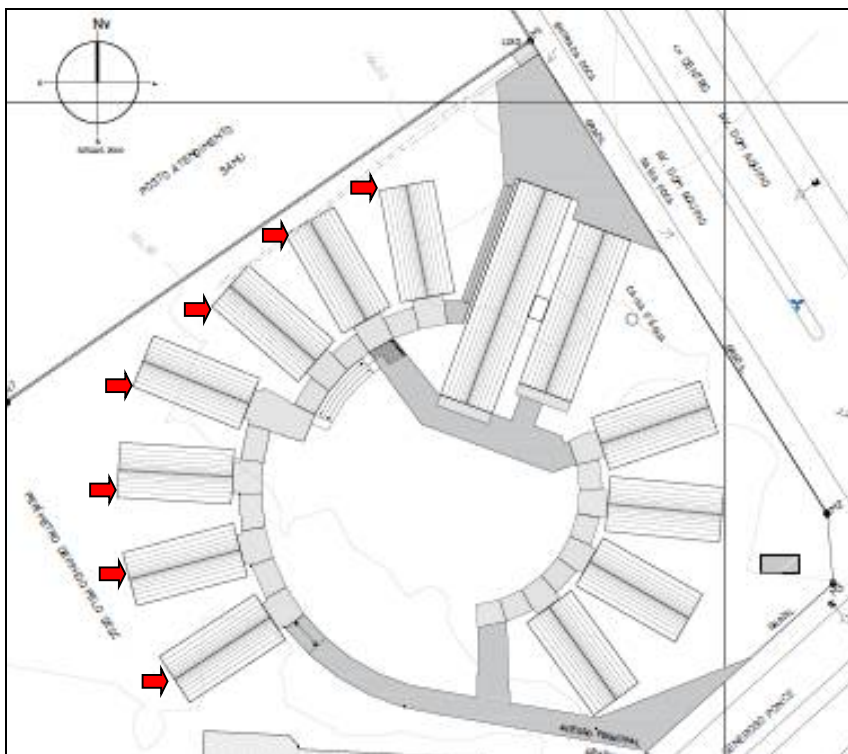
Figura 2 - Layout Geral
