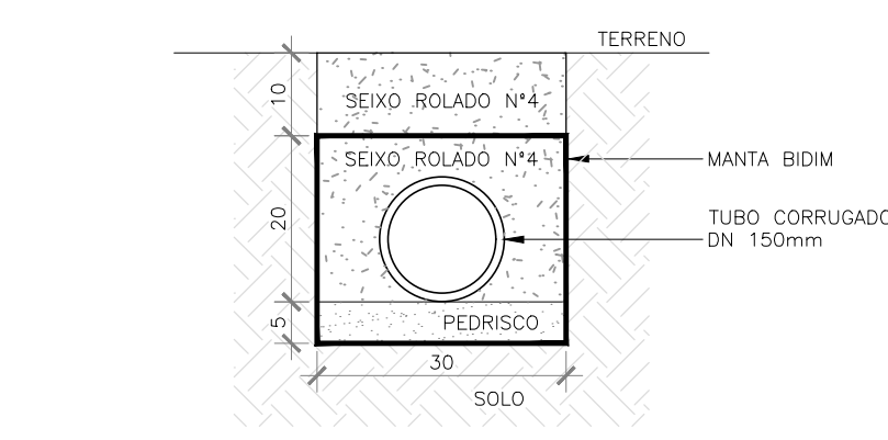
DETALHE DA TRINCHEIRA DRENANTE ESCALA 1:10
