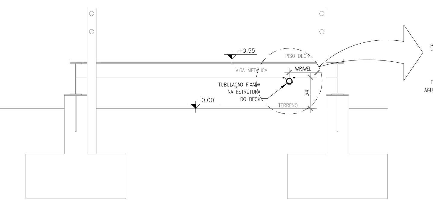
DETALHE DA FIXAÇÃO DAS TUBULAÇÕES SOB DECK SEM ESCALA
