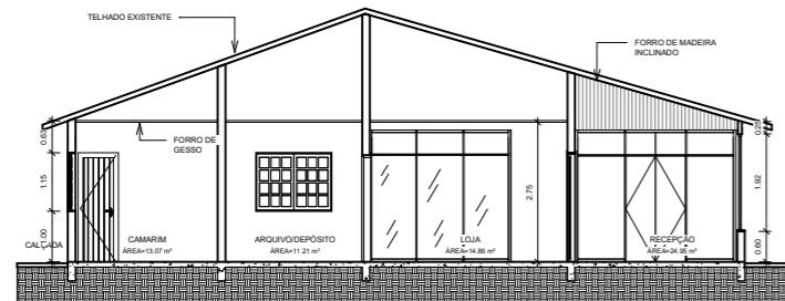
3 Corte A 1: 75
