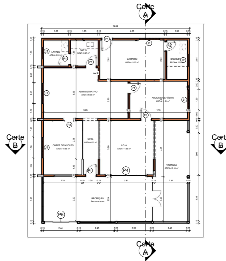
2 PLANTA TÉRREO 1: 75
