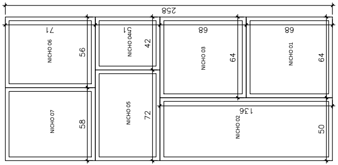
0 VISTA DA PRATELEIRA 1 PARA MONTAGEM
